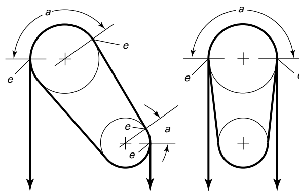
Fig. 8.4.3.1.3 Arc of Contact
