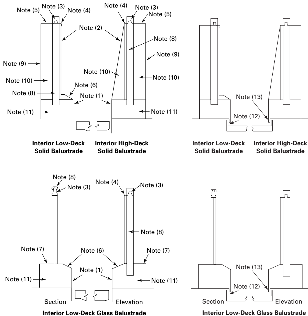
Fig. I-3 Escalator Nomenclature
