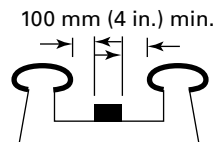
Fig. I-6 Antislip Device (6.1.3.3.12)
